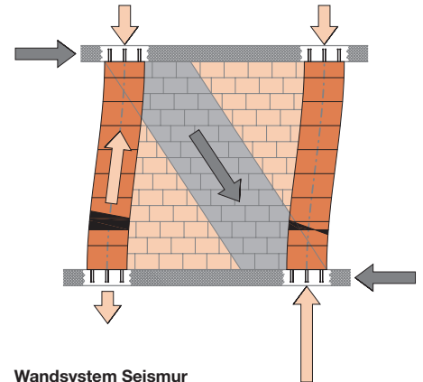
Wandsystem Seismur
